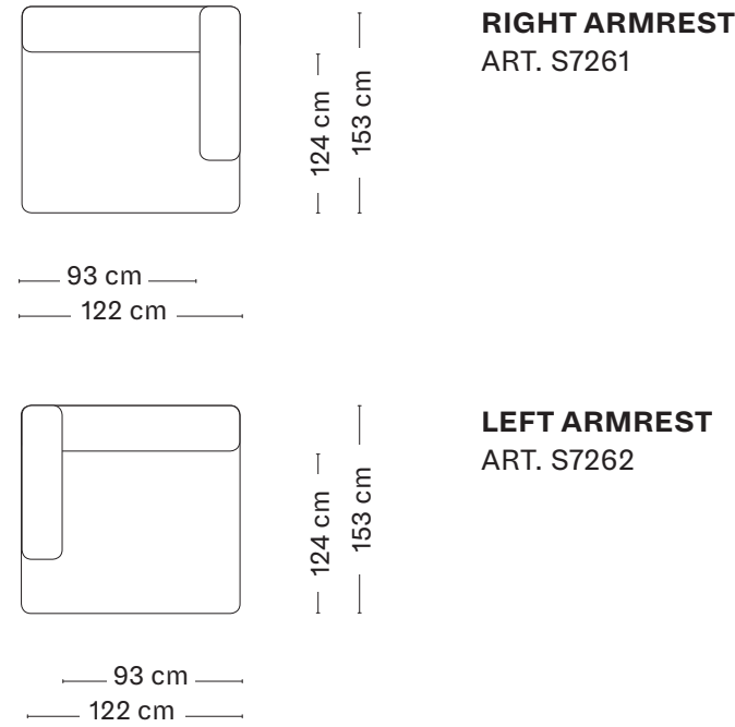
MAGS SOFT WIDE CHAISE LONGUE MODULE LONG
