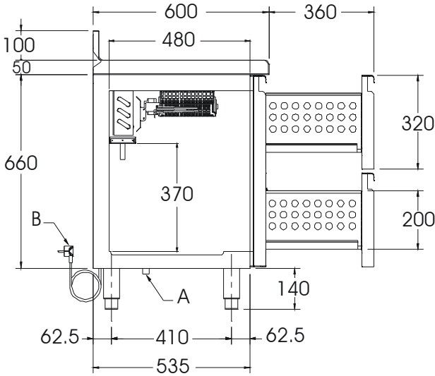
A: Drainpipe Tuyau d'écoulement Abflusrohr B: Power Cable Câble d'alimentation Stromzuführungskabel
