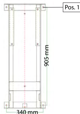
Abbildung 1: Bohrbild für die Montage
