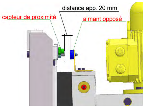
Illustration 6: capteur de proximité et aimant opposé
