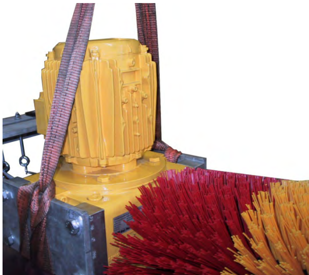
Рисунок 3: Крепление стропа
