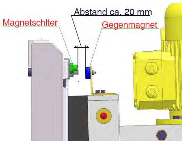
Abbildung 6: Annäherungsschalter und Gegenmagnet
