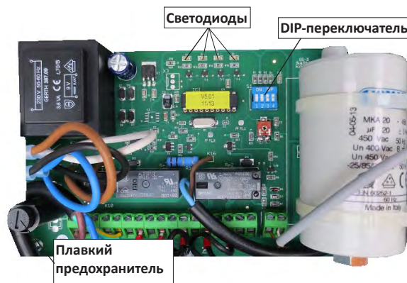
Рисунок 5: Плата управления
