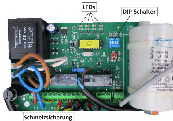
Abbildung 5: Steuerungssplatine
