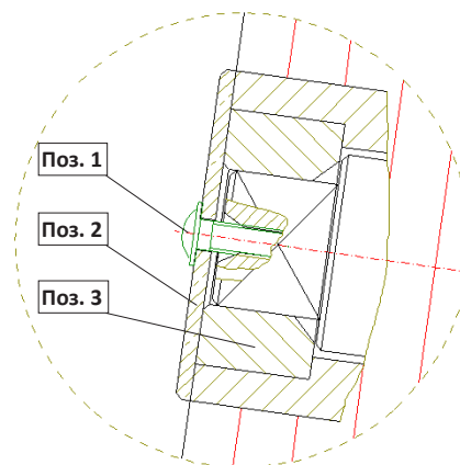
Рисунок 8: Крепление верхней щетки
