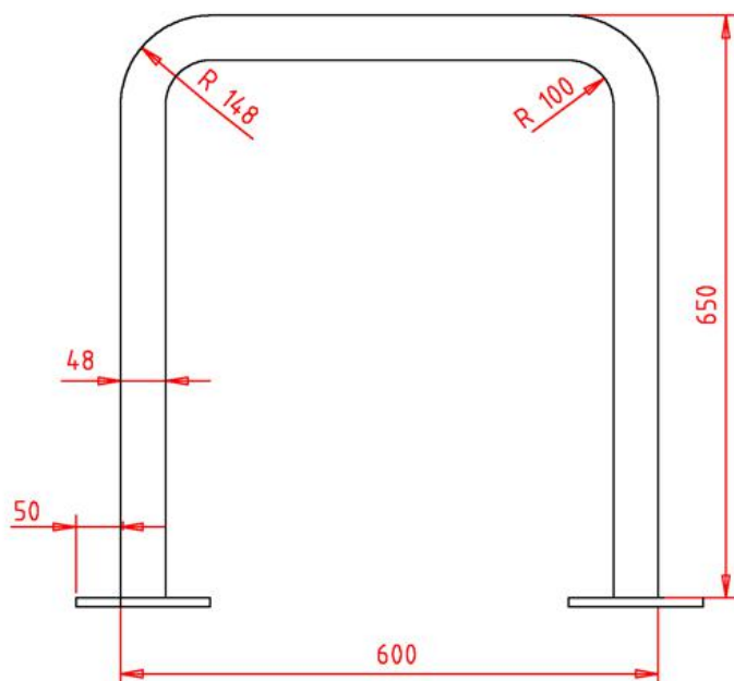
APPUIS VELO / FIETSBEUGEL MODELE A / MODEL A
