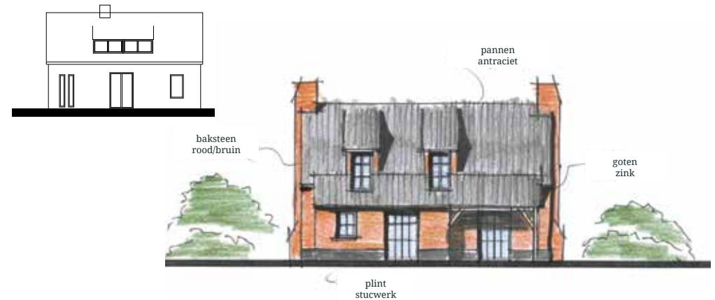
RECHTERGEVEL WEST
