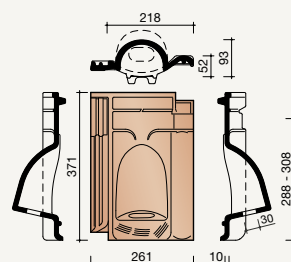
8660 Gierzwaluwp
