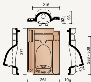
8655 Mussenpan
