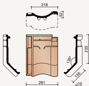
8200 Knikpan*/**
