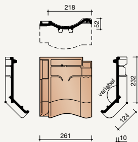
8200 Knikpan op maat (verlijmd)*
