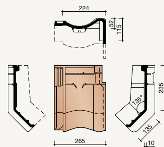
7290 Rechter gevelknikpan**
