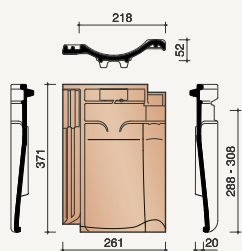
8640 Ventilatie-/haakdoorvoerpan met rooster 25 cm 2
