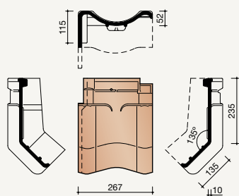
7280 Linker gevelknikpan**
