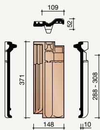
8010 Halve pan
