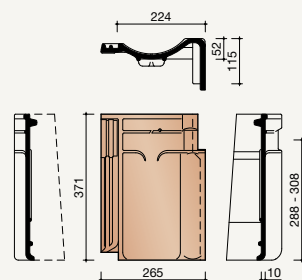
7090 Rechter gevelpan
