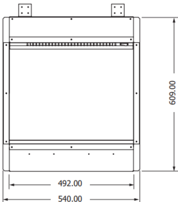
Lijntekening Elektrische haard Club 50e Front
