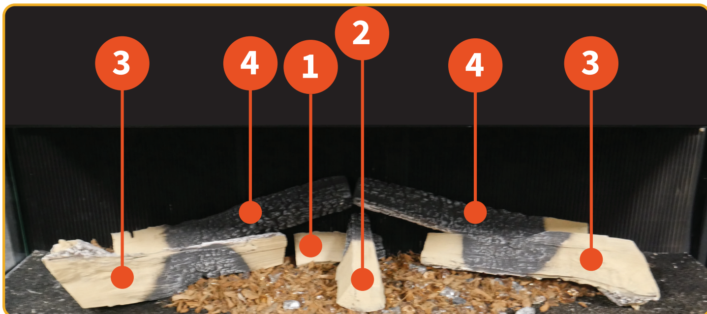
Afb. C.C | Deel 1 van de plaatsing van de stammen
