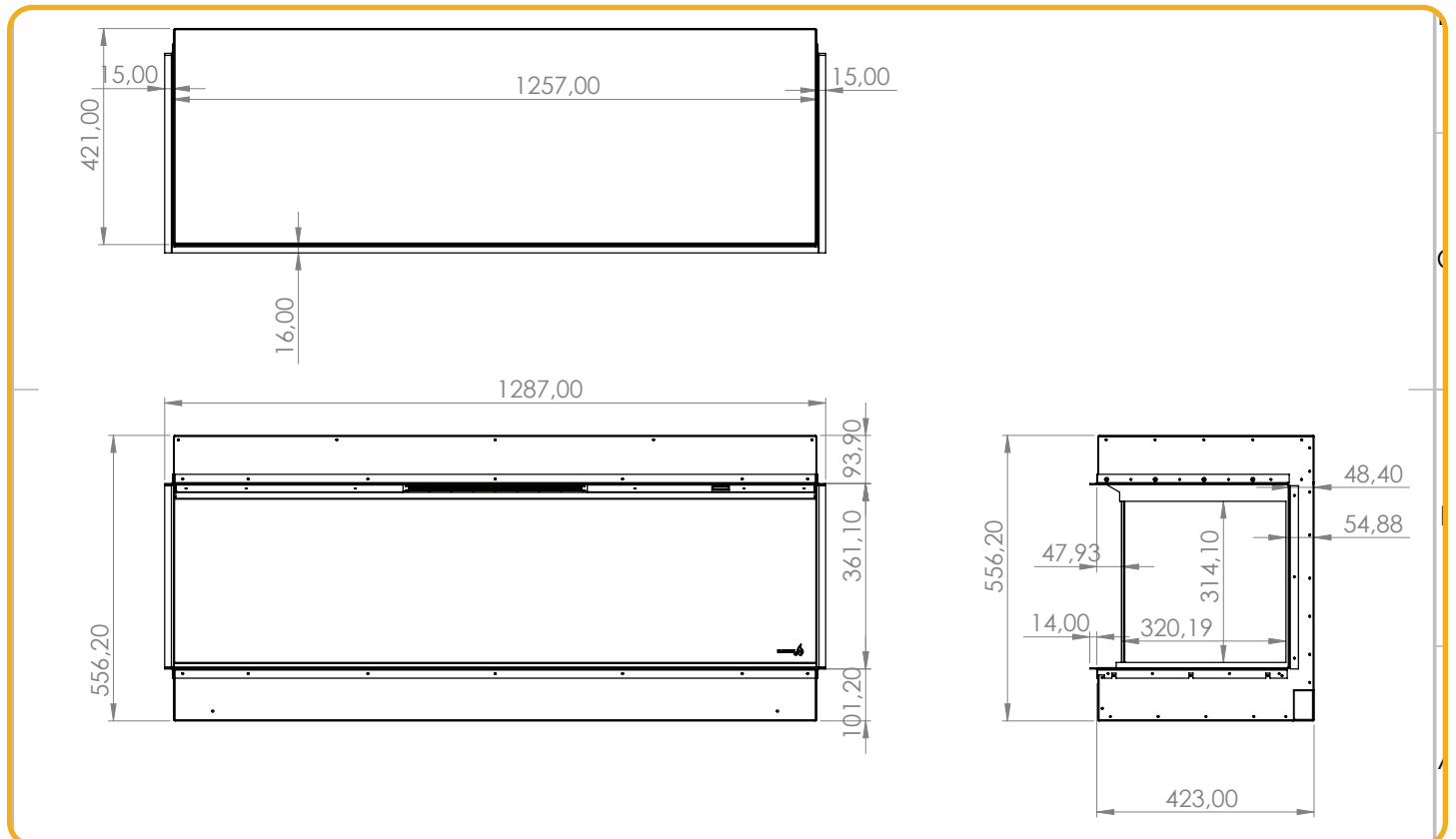
Afb. B.A | Ambiance 125-E 3S maten
