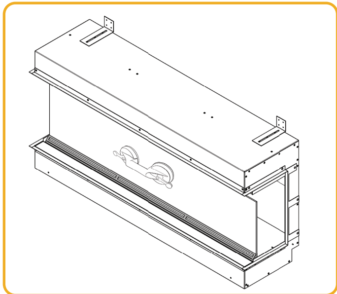
Afb. 9.1 | Plaats onderrand van effect glas
