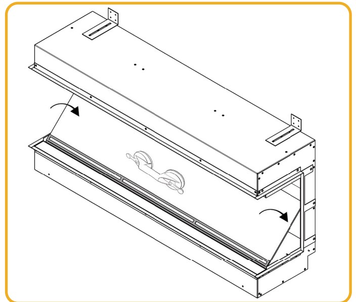
Afb. 9.2 | Kantel het effect glas naar binnen
