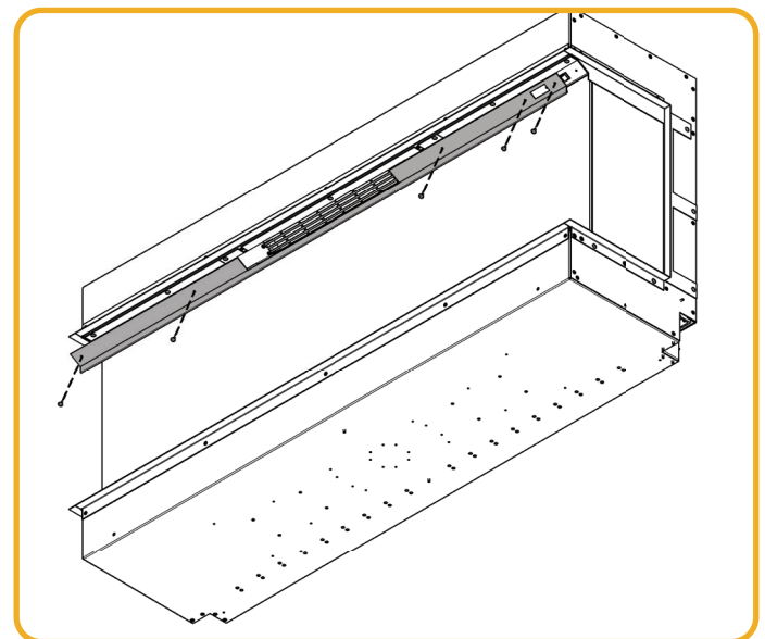
Afb. 9.4 | MOnteer de opsluit beugel
