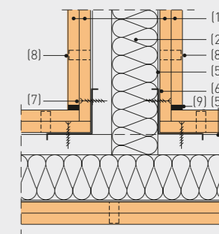
Wandaansluiting in T-vorm met onderbroken langszijde en L-binnenhoekprofiel
