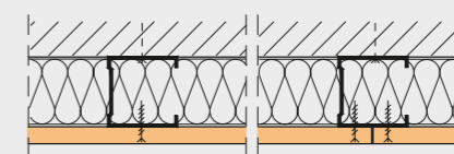
Onderconstructie van CW-profielen, bevestiging met schroeven aan achterwand, enkel beplaat
