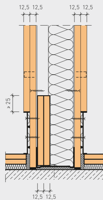
Achterliggende plint 90 min. (maten in mm)
