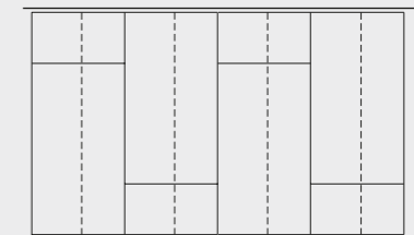
Plaats van de voegen bij enkele fermacell beplating
