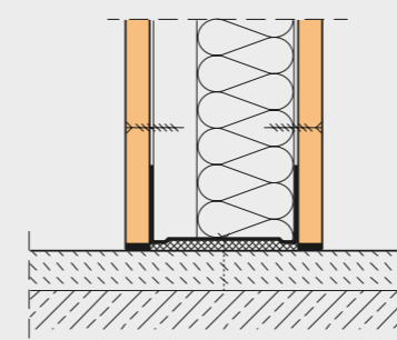
Scheidingswand op zandcement afwerkvloer
