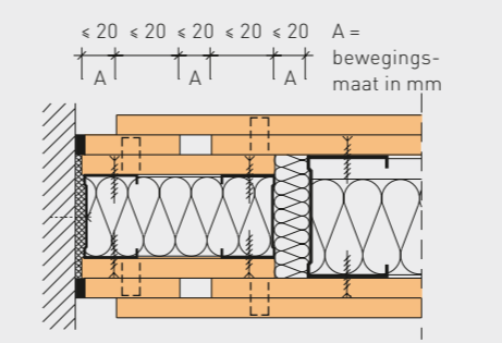
fermacell montagewand, dubbel beplaat, 90 min. Glijdende wand- en/of gevelaansluiting met twee CW-profielen en plaatstroken
