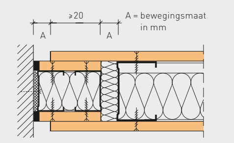
fermacell montagewand, enkel beplaat, 30 min./60 min. Glijdende wand- en/of gevelaansluiting met twee CW-profielen en plaatstroken
