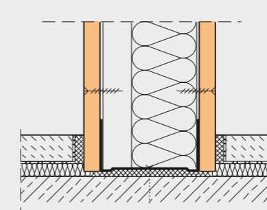
Zwevende afwerkvloer tegen scheidingswand
