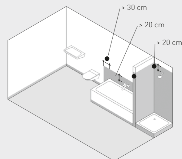
Wand-hoekaansluiting in sproeibereik badkamer met badkuip en douchecel
