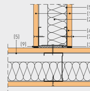
Wandaansluiting in T-vorm, CW-profiel in CW-profiel geschroefd
