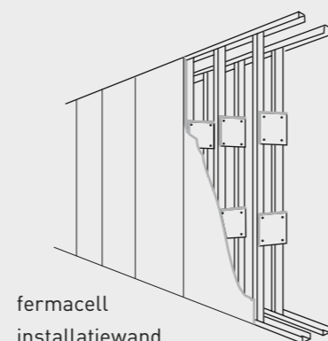
Verbinding van de twee onderconstructies bij een fermacell installatiewand
