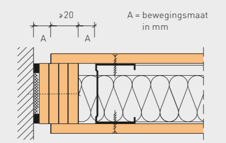
fermacell montagewand, enkel beplaat, 30 min./60 min. Glijdende wand- en/of gevelaansluiting met strokenbundel
