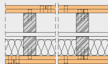
fermacell montagewand met spouwisolatie als dubbele staanderwand, dubbel beplaat
