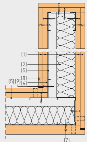
Hoekaansluitingen bij enkele en dubbele beplating
