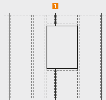
Detail 2: raamopening, platen gevlagd
