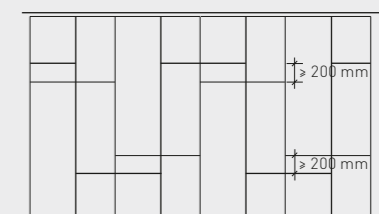
Plaats van de voegen bij dubbele fermacell beplating
