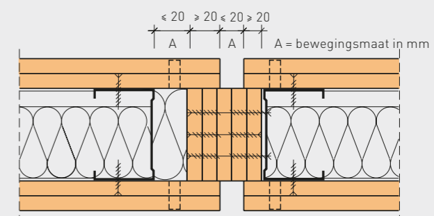
fermacell montagewand, dubbel beplaat, 90 min. Dilatatievoeg met strokenbundel
