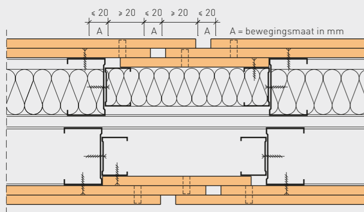
fermacell montagewand als dubbele staanderwand, dubbel beplaat, 90 min. Dilatatatievoeg met plaatstroken
