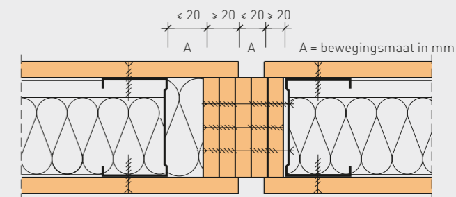
fermacell montagewand, enkel beplaat, 30 min./60 min. Dilatatievoeg met strokenbundel
