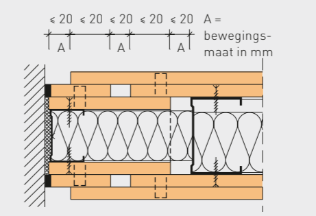
fermacell montagewand, dubbel beplaat, 90 min. Glijdende wand- en/of gevelaansluiting met een CW-profiel en plaatstrook
