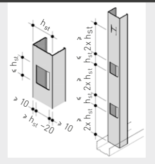
Maximale uitsnijdingen in CW-profielen van metalen systeemwanden (ter plaatse gebouwd)
