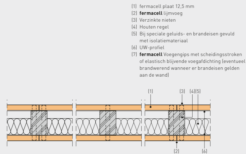
fermacell montagewand met stalen/houten onderconstructie
