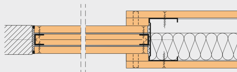
Reduceeraansluiting van een enkele staanderwand met loodvulling 2,5 mm
