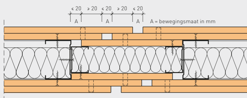
fermacell montagewand, dubbel beplaat, 90 min. Dilatatievoeg met plaatstroken
