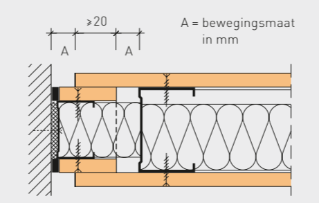
fermacell montagewand, enkel beplaat, 30 min./60 min. Glijdende wand- en/of gevelaansluiting met een CW-profiel en plaatstrook
