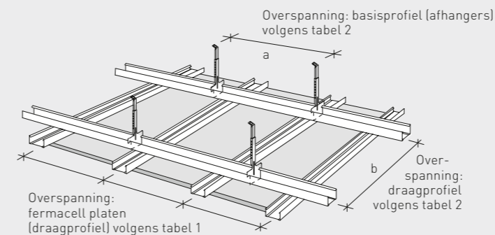
Verlaagd plafond met metalen onderconstructie, afgehangen
