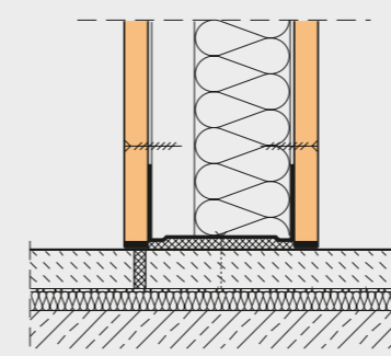
Scheidingswand op zwevende afwerkvloer met scheidingsvoeg
