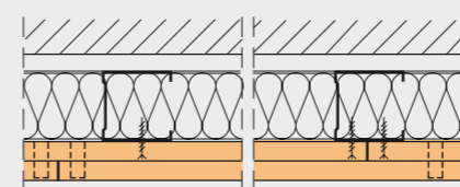
fermacell voorzetwand, enkel beplaat
