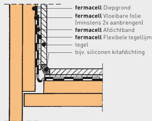
Wand-hoekaansluiting in sproeibereik
