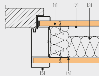
(1) fermacell afbouwplaat (2) UW-profiel (3) Minerale wol (4) CW-profiel
