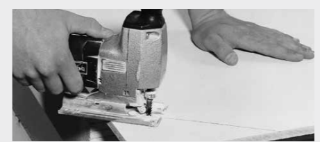
Zagen met decoupeerzaag met variabel toerental
