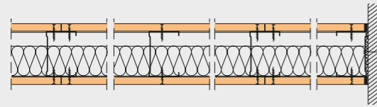
Plaatsing van de fermacell Gipsvezelplaten op metalen onderconstructie
