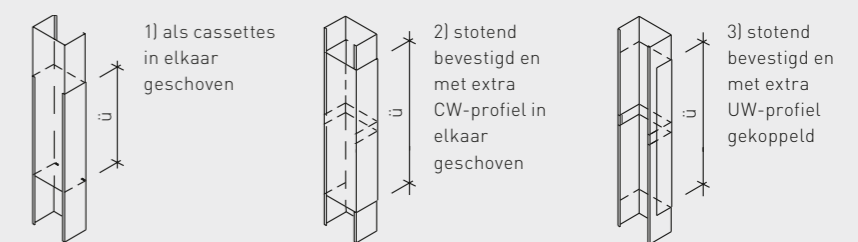
Mogelijkheden voor verlenging van twee CW-profielen
