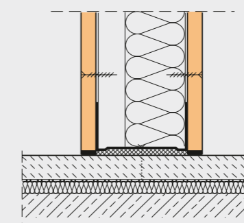
Scheidingswand op doorlopende zwevende afwerkvloer
