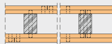
fermacell montagewand zonder spouwisolatie als enkele staanderwand, dubbel beplaat
