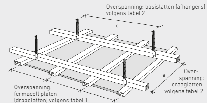
Verlaagd plafond met houten onderconstructie, afgehangen
