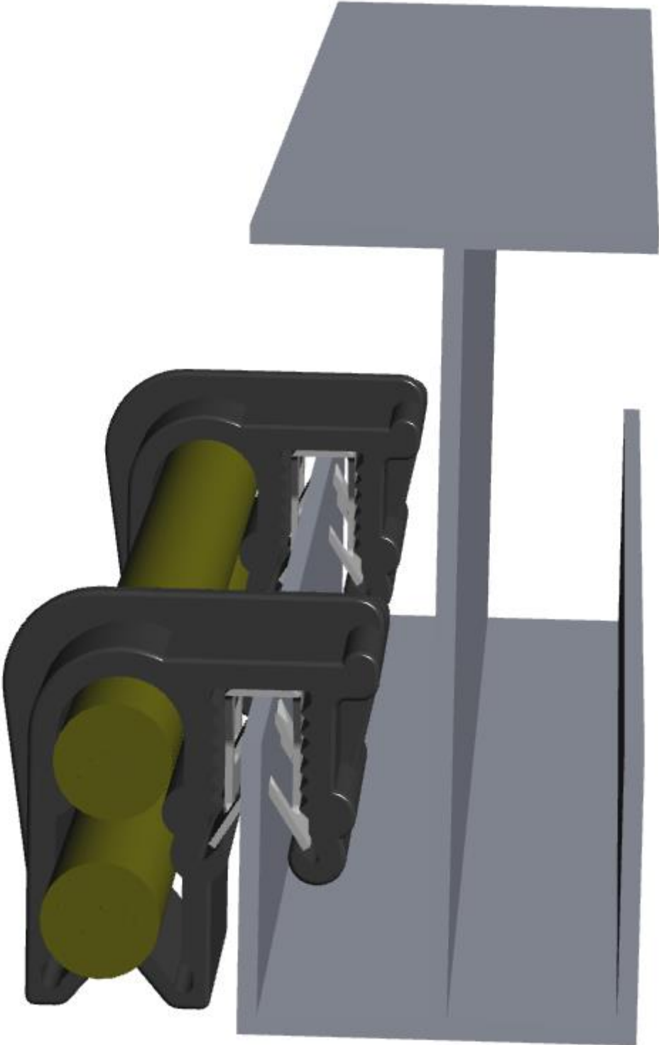
Figuur 1. 3D-view van de kabelklem
