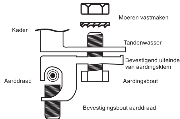
Figuur 10 Aardingsmethode van de PV-module
