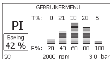
Afb. 16: weergave van het vermogenshistogram
