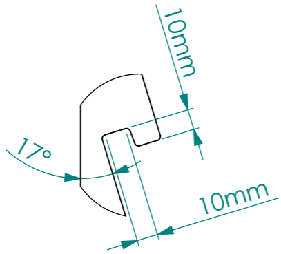
DÉTAIL X ECHELLE 2 : 5
