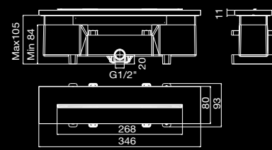
60 C400 ●●●●●●●●●● Rociador cascada empotrado a pared inox 350 mm Waterfall concealed inox showerhead wall mounted 350 mm встроенная душевая лейка нержавеющей эффект каскада 350 мм
