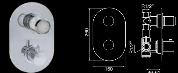
77 601 / 77 602 / 77 603 ●●●●● Termostático baño ducha empotrar con inversor 1/2/3 vías Thermostatic concealed bath shower with diverter 1/2/3 ways Mitigeur thermostatique bain/douche à encastrer avec inverseur 1/2/3 vois Thermostat für brause/wannenbatterie mit umstellung 1/2/3 abgängen Термостатический смеситель встроенный душ и ванна на 1/2/3 выхода
