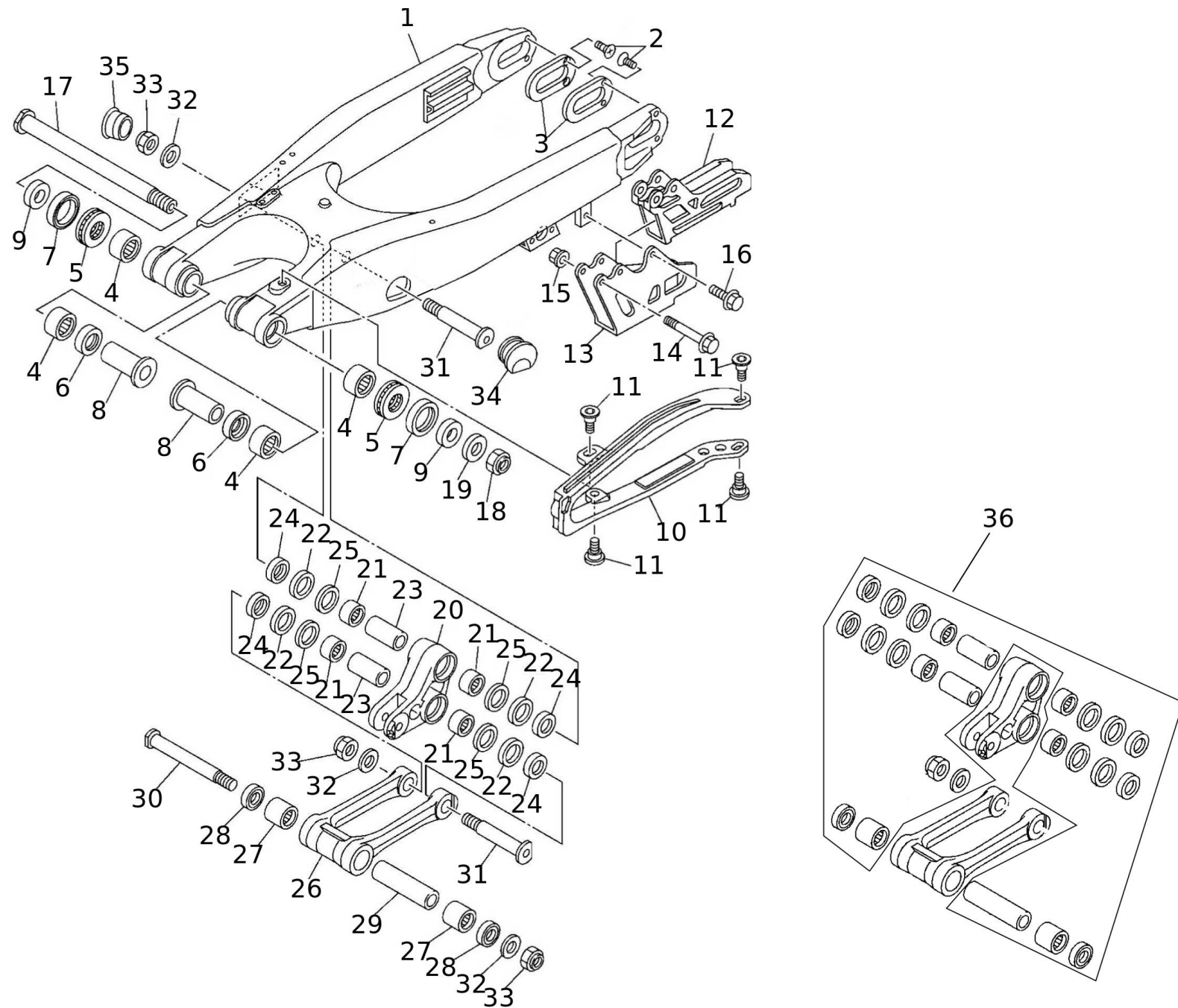
Schwinge
