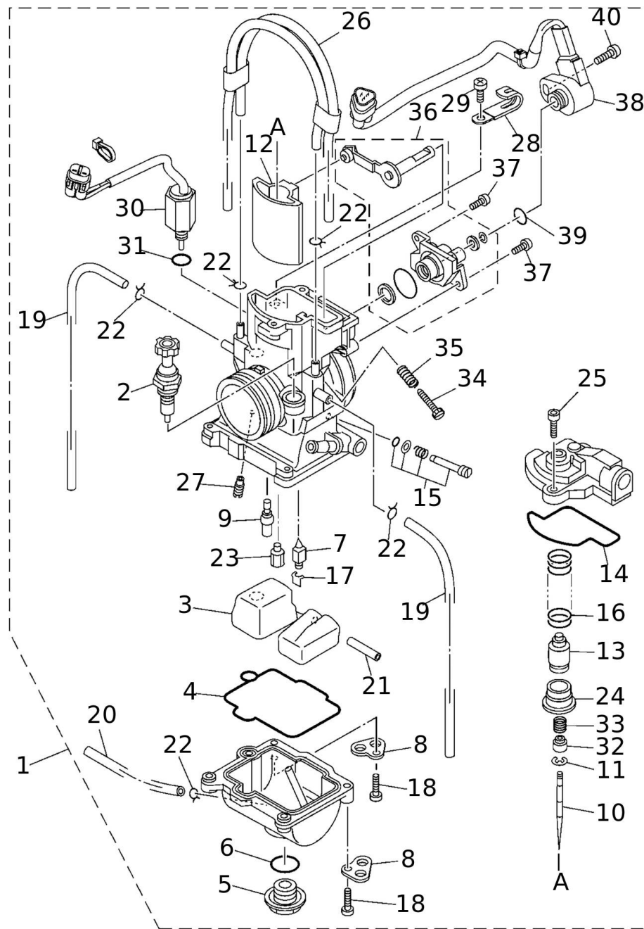
Vergaser
