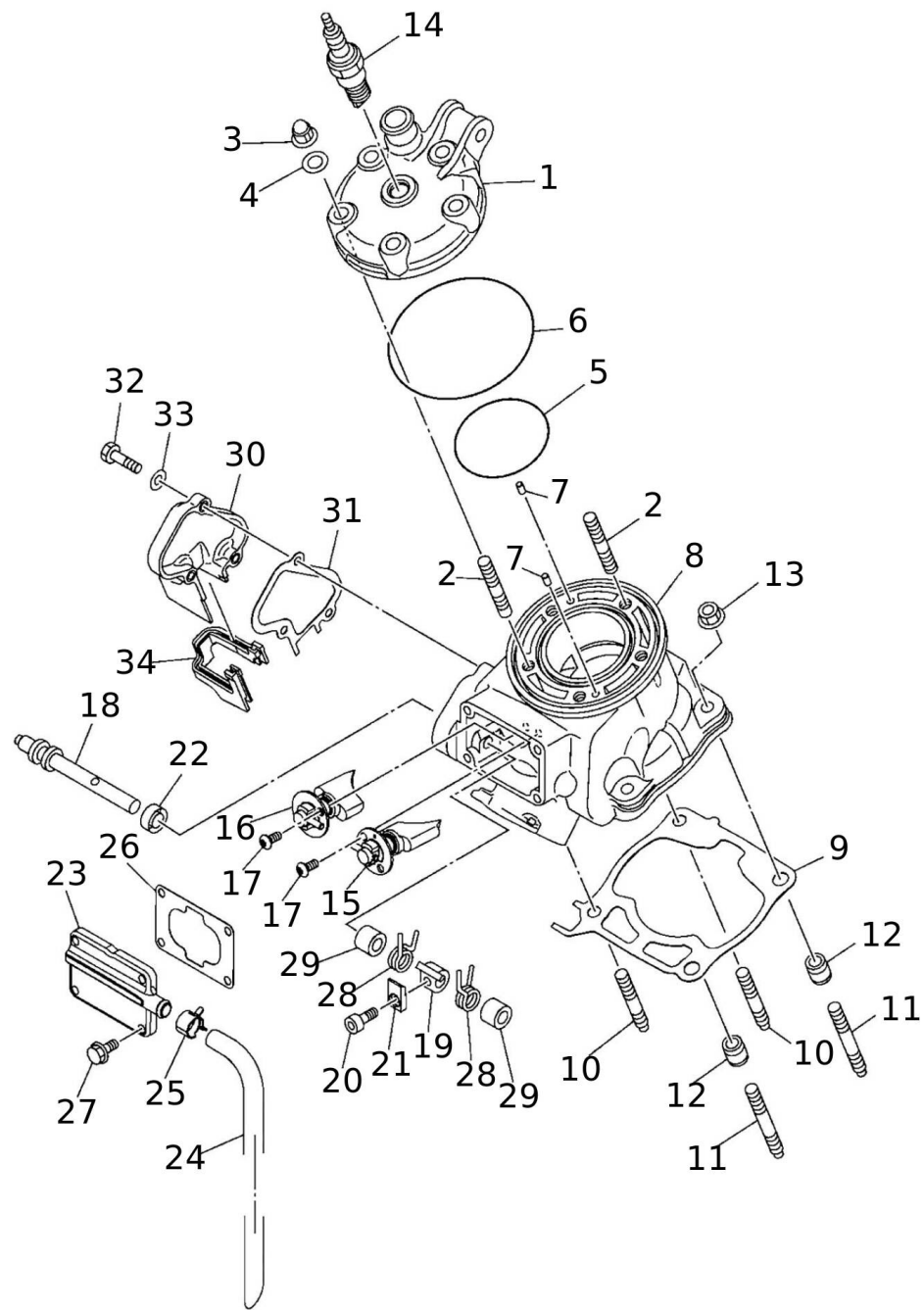
Kopf - Zylinder
