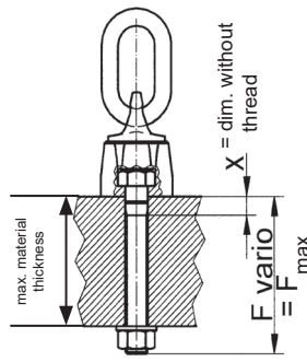
Pic. 8: VWBG-V (Vario)
