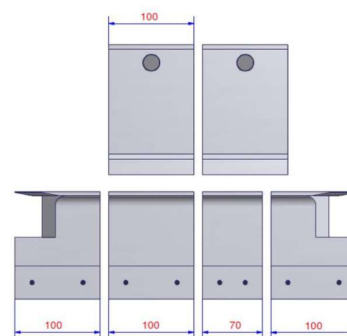
Fensterbankeinsatz Variabel
