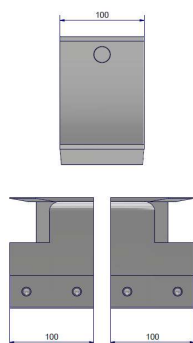
Fensterbankeinsatz Standard
