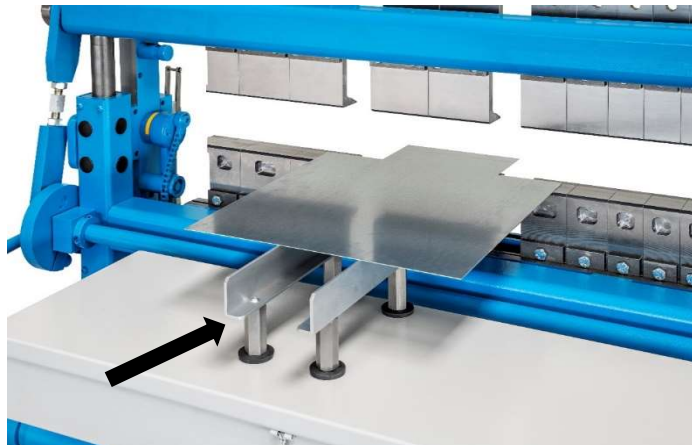
Werkstückauflage
