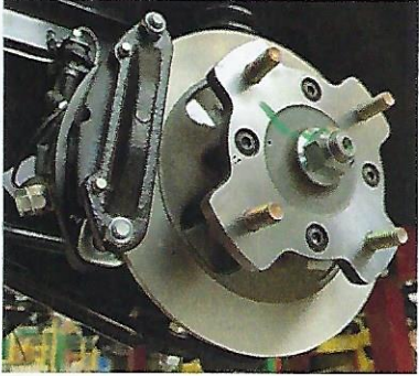
Rondom schijfremmen
