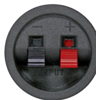
Typ A: Rund Einpress-Montage Maße: \varnothing 56,5 mm Lochkreisausschnitt 45 mm Einbautiefe ca. 24 mm
