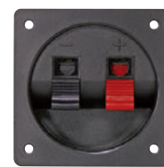
Typ B: Eckig Schraubbefestigung Maße 57 x 57 mm, Einbautiefe ca. 23 mm
