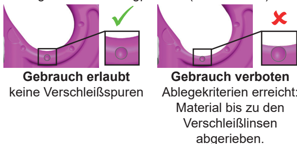
Abb. 2: Verschleißlinsen
