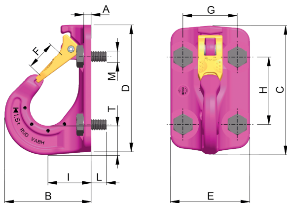
Abb. 3: Bemaßung
