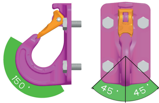
Abb. 1: Zulässige Belastungsrichtungen
