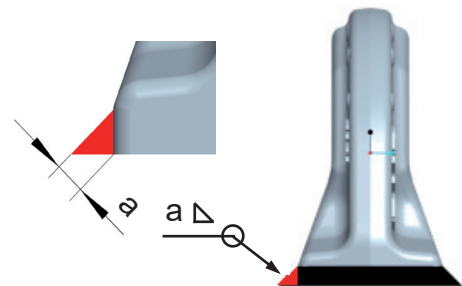
Abb. 6: Schweißnahtanordnung
