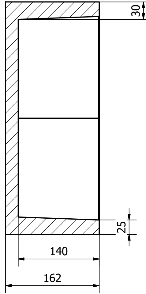
A-A ( 1 : 4 )
