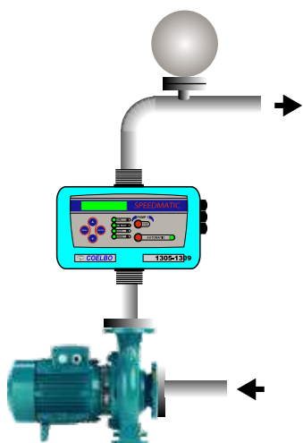
fig.1a. Assemblage individuel.
