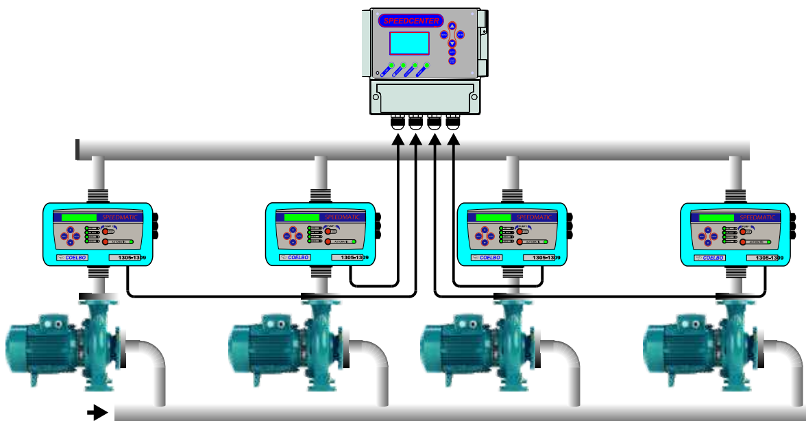
fig.1c. Montaje en grupos de 3 o 4 bombas en régimen MASTER-SLAVE a través de Speedcenter.
