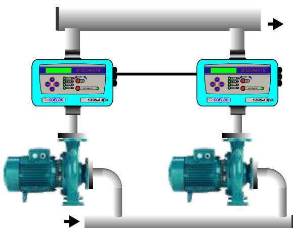
fig.1b. Montaje en grupos de 2 bombas en régimen MASTER-SLAVE.
