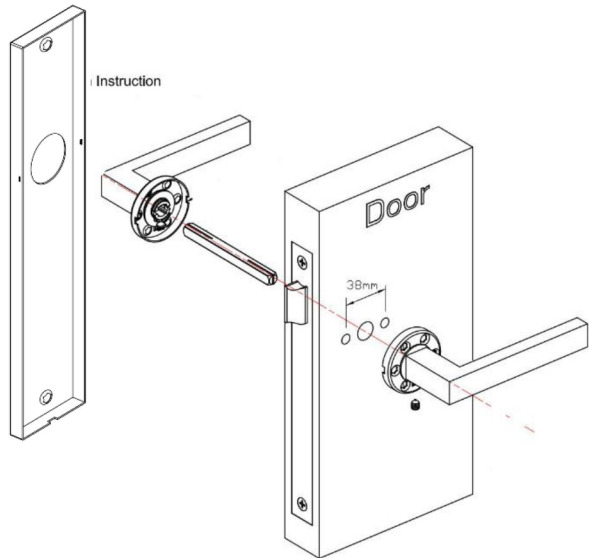
Afb.2 Montagevolgorde
