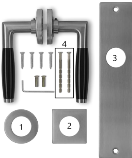
Afb.1 Onderdelen
