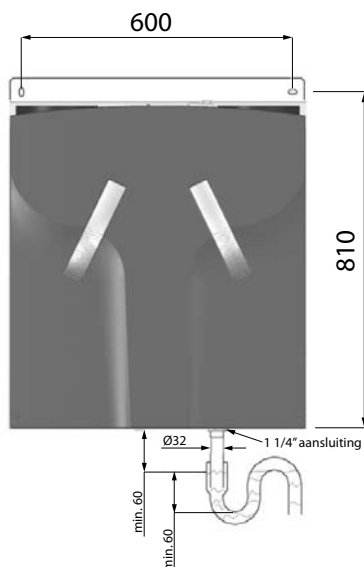
WHR 950/960 - RECHTS
