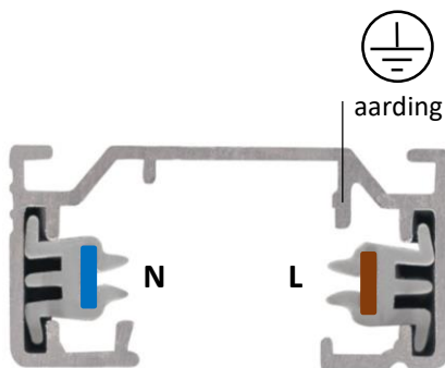
Doorsnede rails
