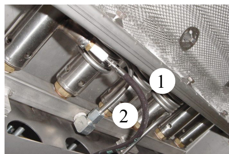
Afb. 4-6: Verdampers
