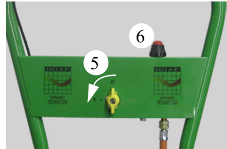
Afb. 5-4: Openen machine-gaskraan
