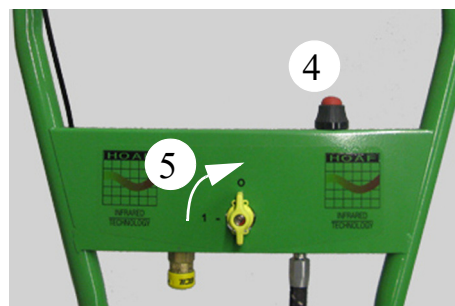
Afb. 5-22: Machine-gaskraan sluiten
