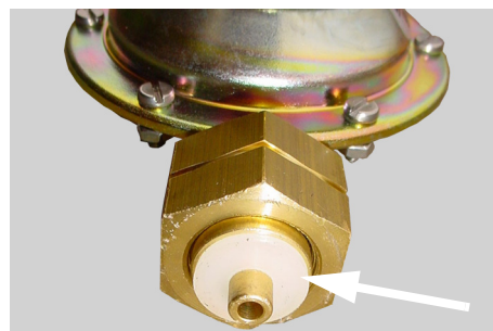
Afb. 3-3: Afsluitring
