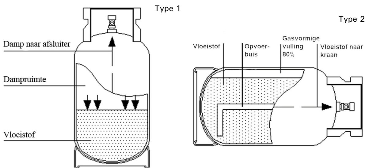
Afb. 6-1: Gasflessen
