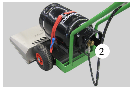
Afb. 5-7: Openen gasfles
