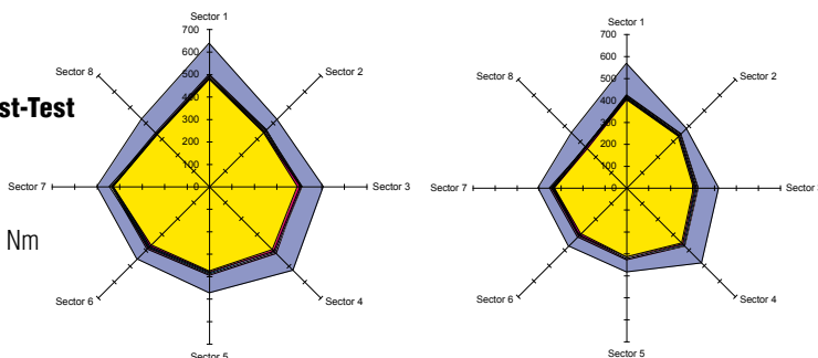
Abb. 1: Höhere Dauerspannkraft dank neuer Gehäusekonstruktion.
