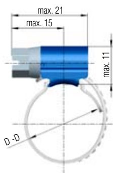
Die Abmessungen entsprechen den Spannbereichen 8-14 bis 25-40*
