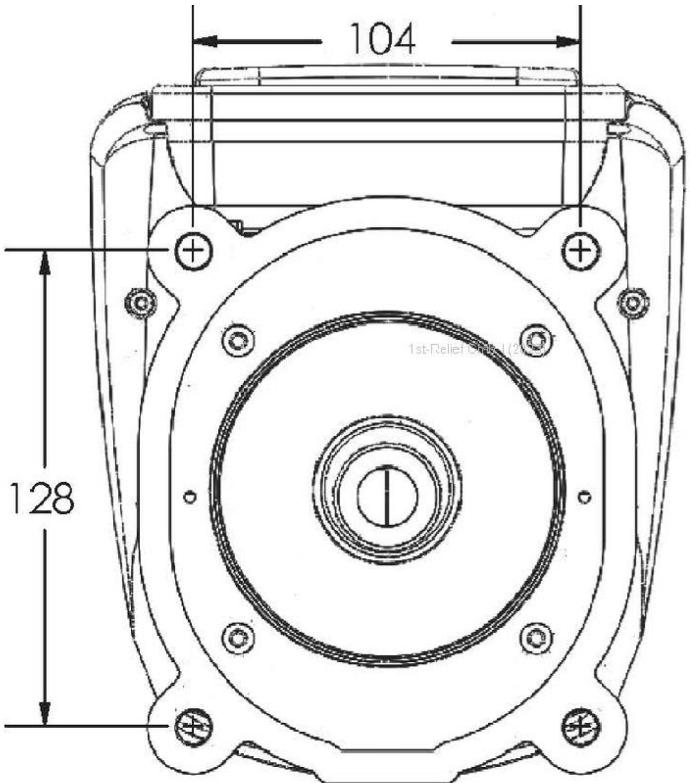
Figure 1 LED Suchscheinwerfer Grundplatte
