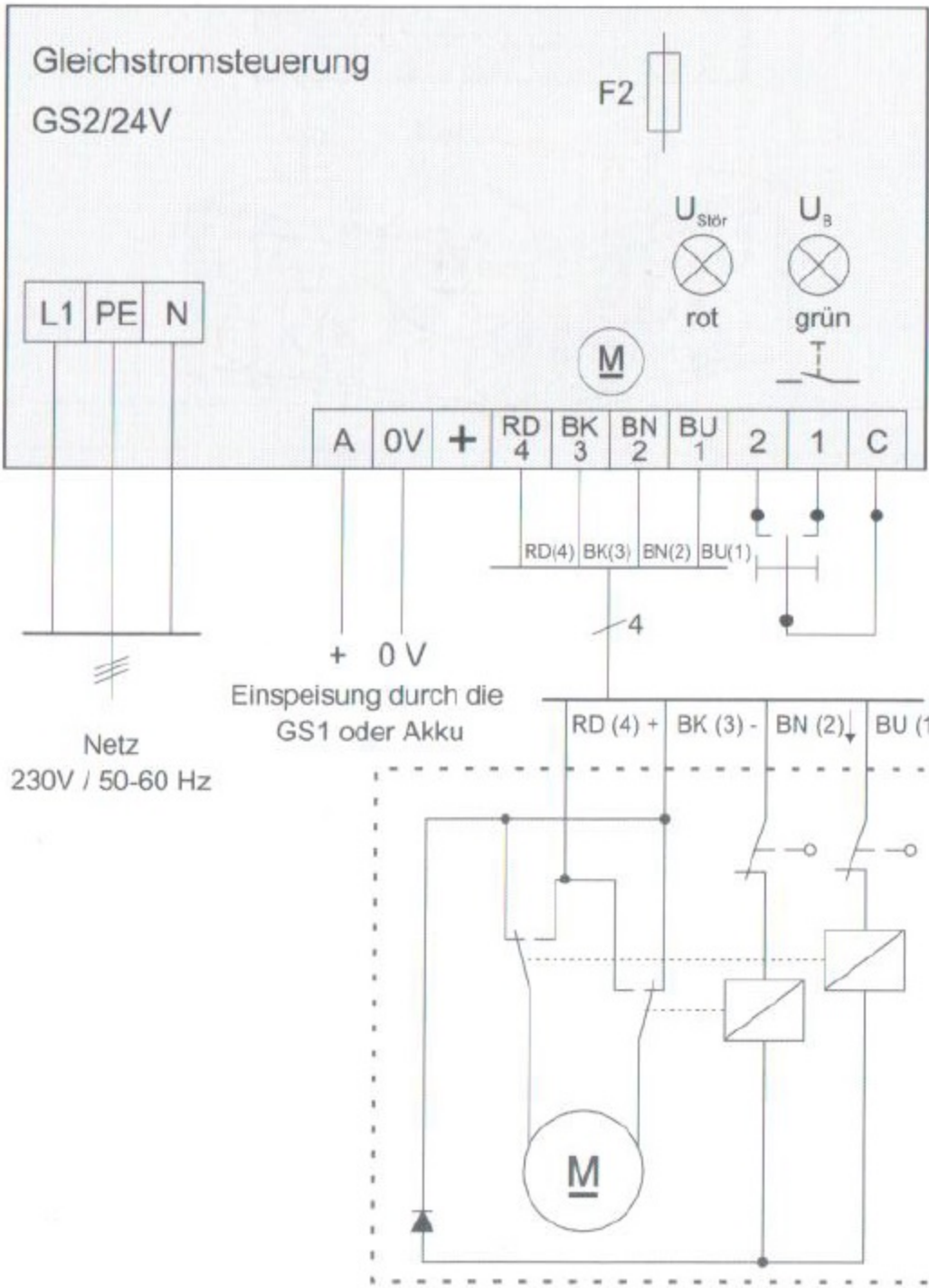
Gleichstromrohrantrieb 24 V
