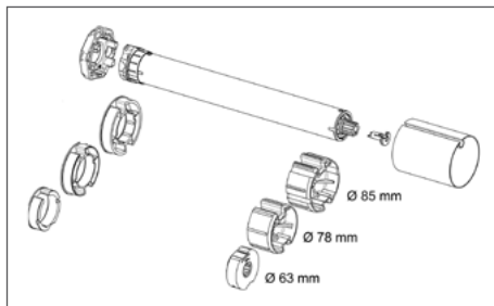
Bild 1: Beispiele für verschiedene Wellengrößen Bild 2: Kupplungssicherung*
