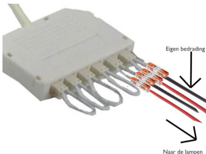
Figuur 3: Verdeelblok
