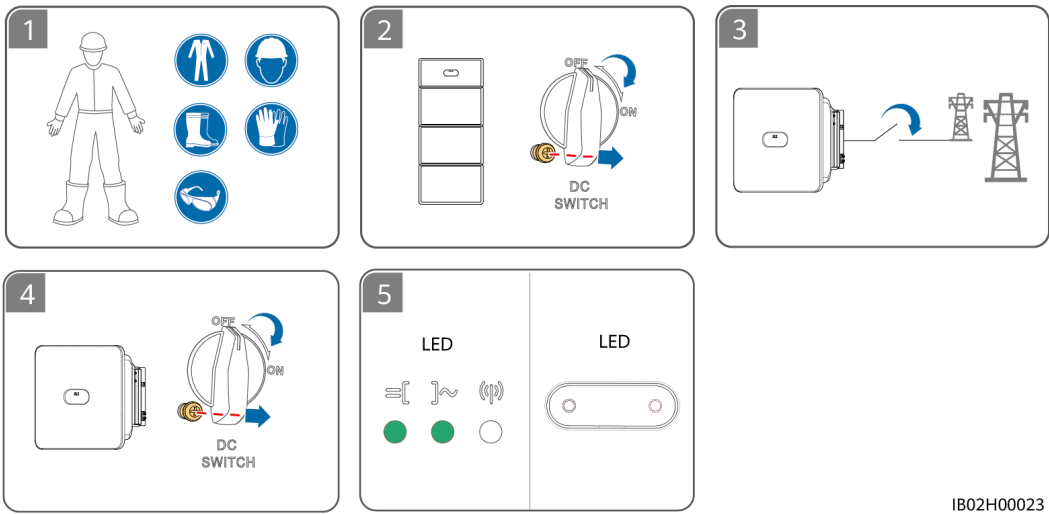
Afbeelding6-1 Inschakelproces
