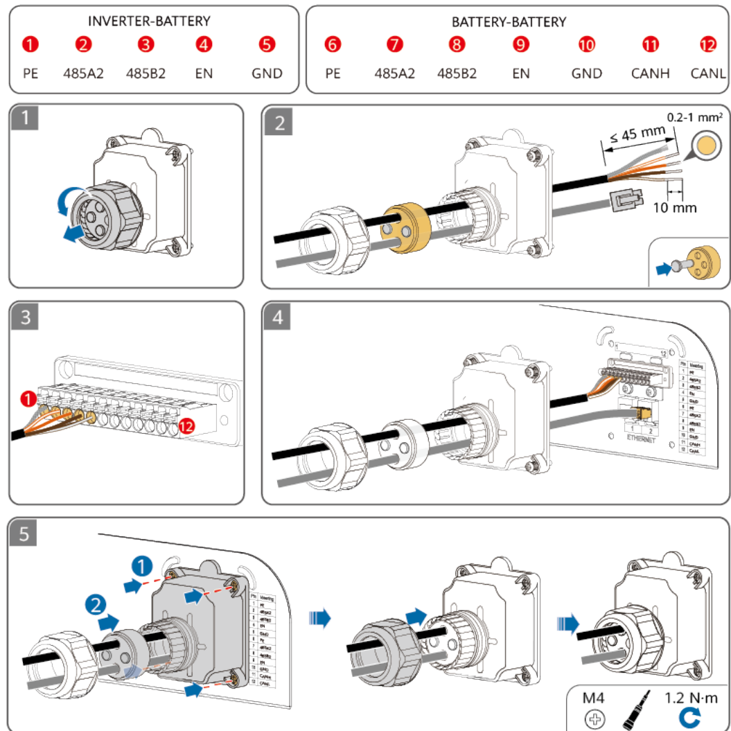
Afbeelding5-7 Signaalpoort aansluitingen
