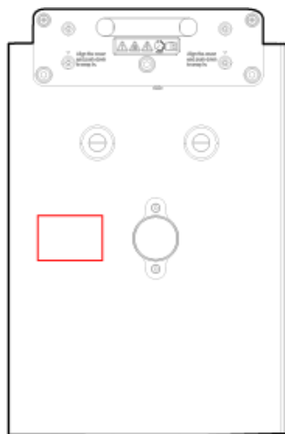
Afbeelding2-16 Positie van het typeplaatje van de Energieopslagmodules
