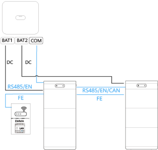
Afbeelding2-10 De ESS'en aansluiten op de omvormer (2)
