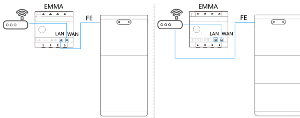
Afbeelding5-8 Netwerkpoort aangesloten op de EMMA of router
