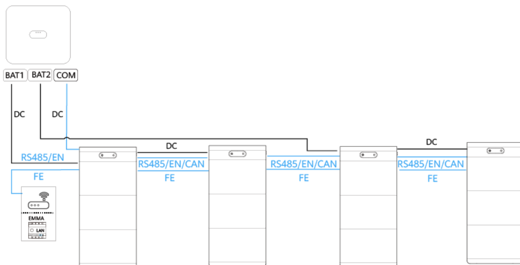
Afbeelding2-12 De ESS'en aansluiten op de omvormer (4)
