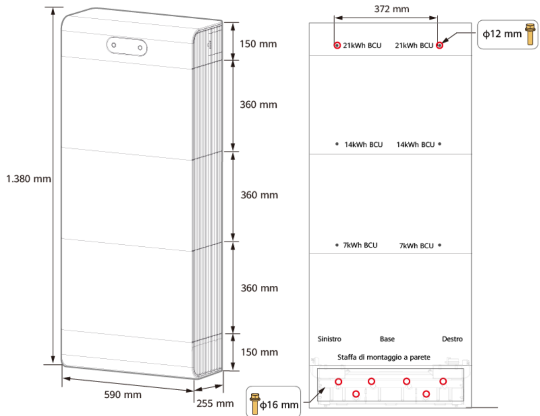
Afbeelding4-5 Afmetingen voor wandmontage
