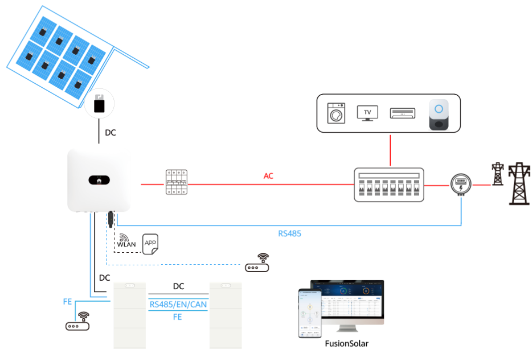
Afbeelding2-7 Via het net-scenario
