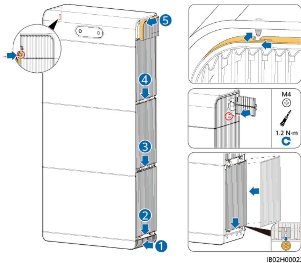
Afbeelding5-12 Decoratieve hoezen plaatsen
