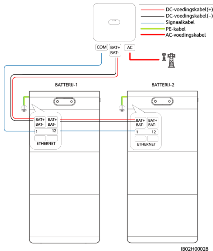
Afbeelding3-1 Kabelaansluitschema
