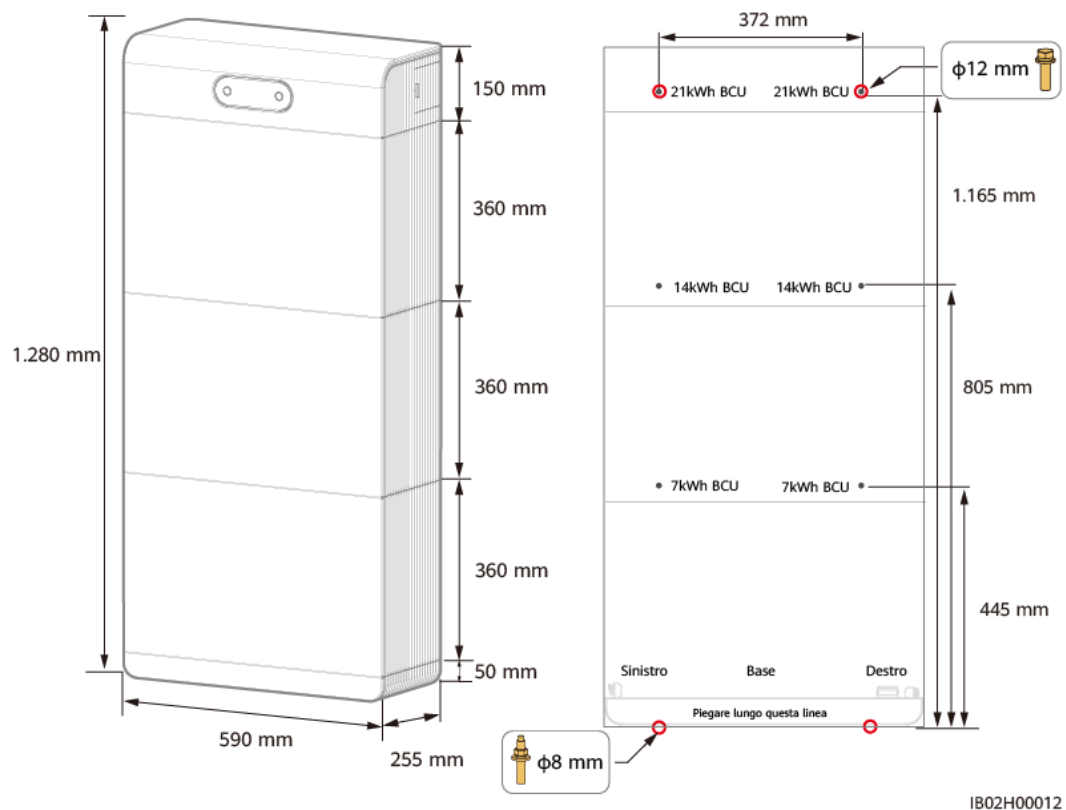
Afbeelding4-4 Afmetingen voor vloermontage
