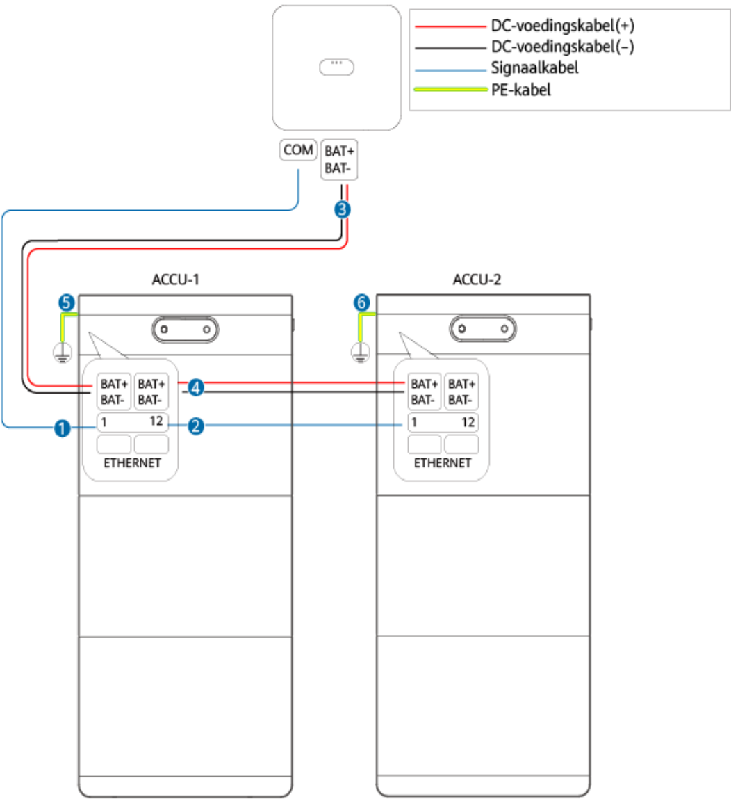
Afbeelding5-1 ESS-kabelaansluitingen
