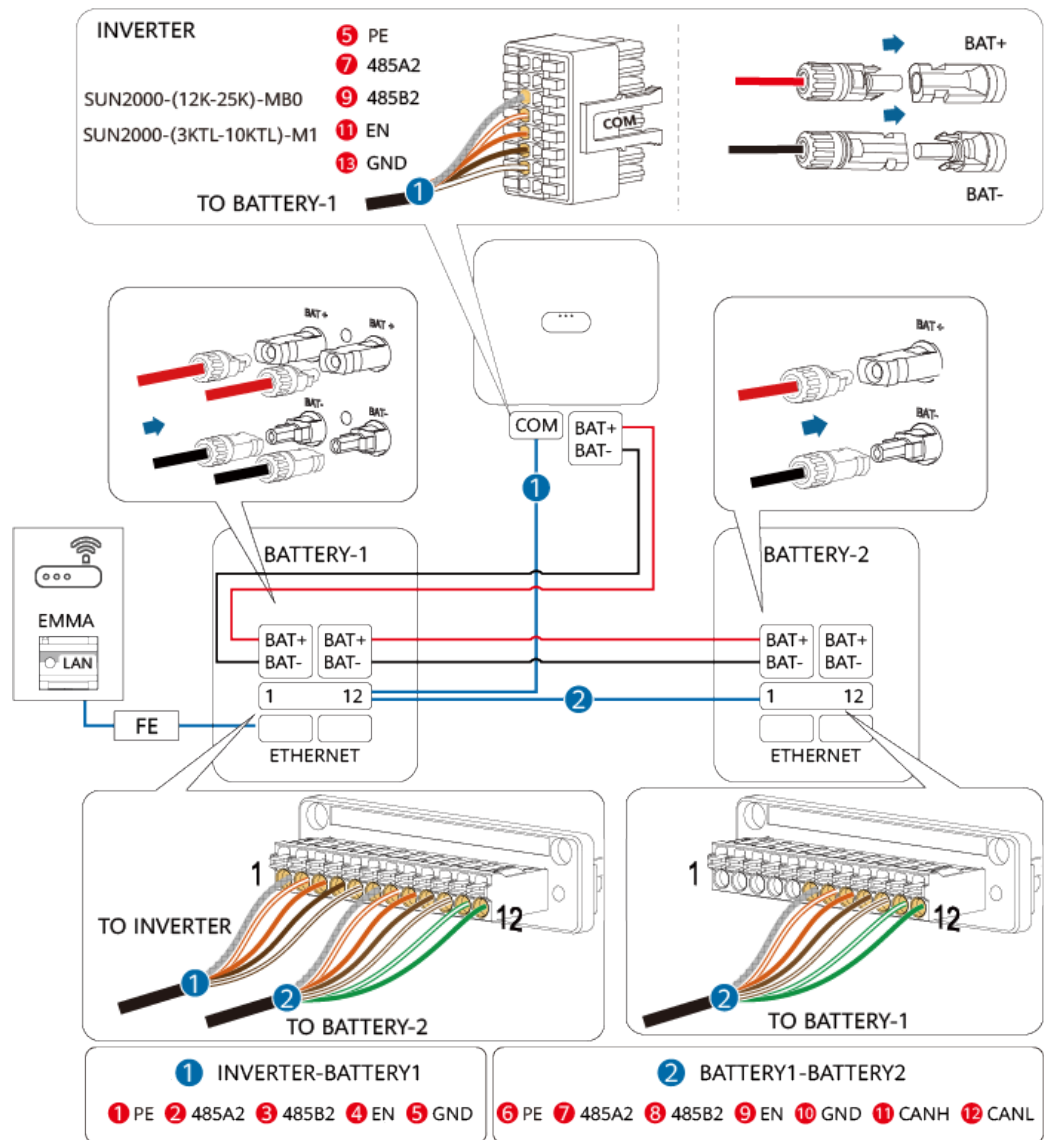
Afbeelding5-9 Omvormer aangesloten op twee ESS'en
