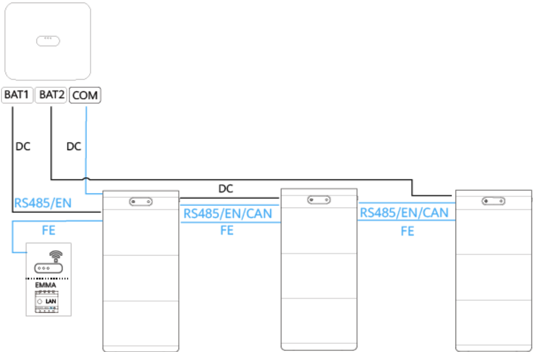
Afbeelding2-11 De ESS'en aansluiten op de omvormer (3)
