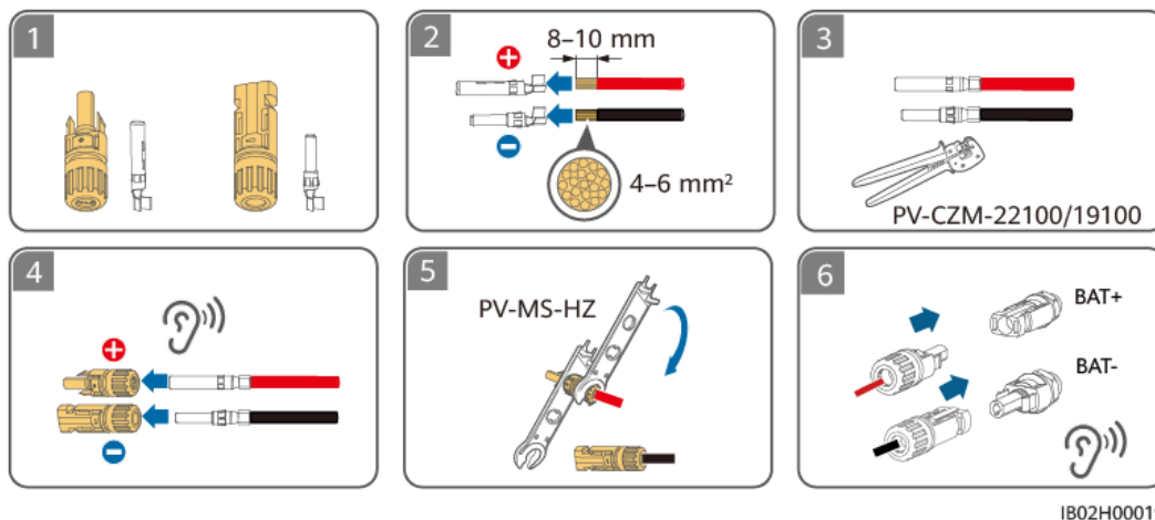
Afbeelding5-4 De DC-ingangskabels aansluiten
