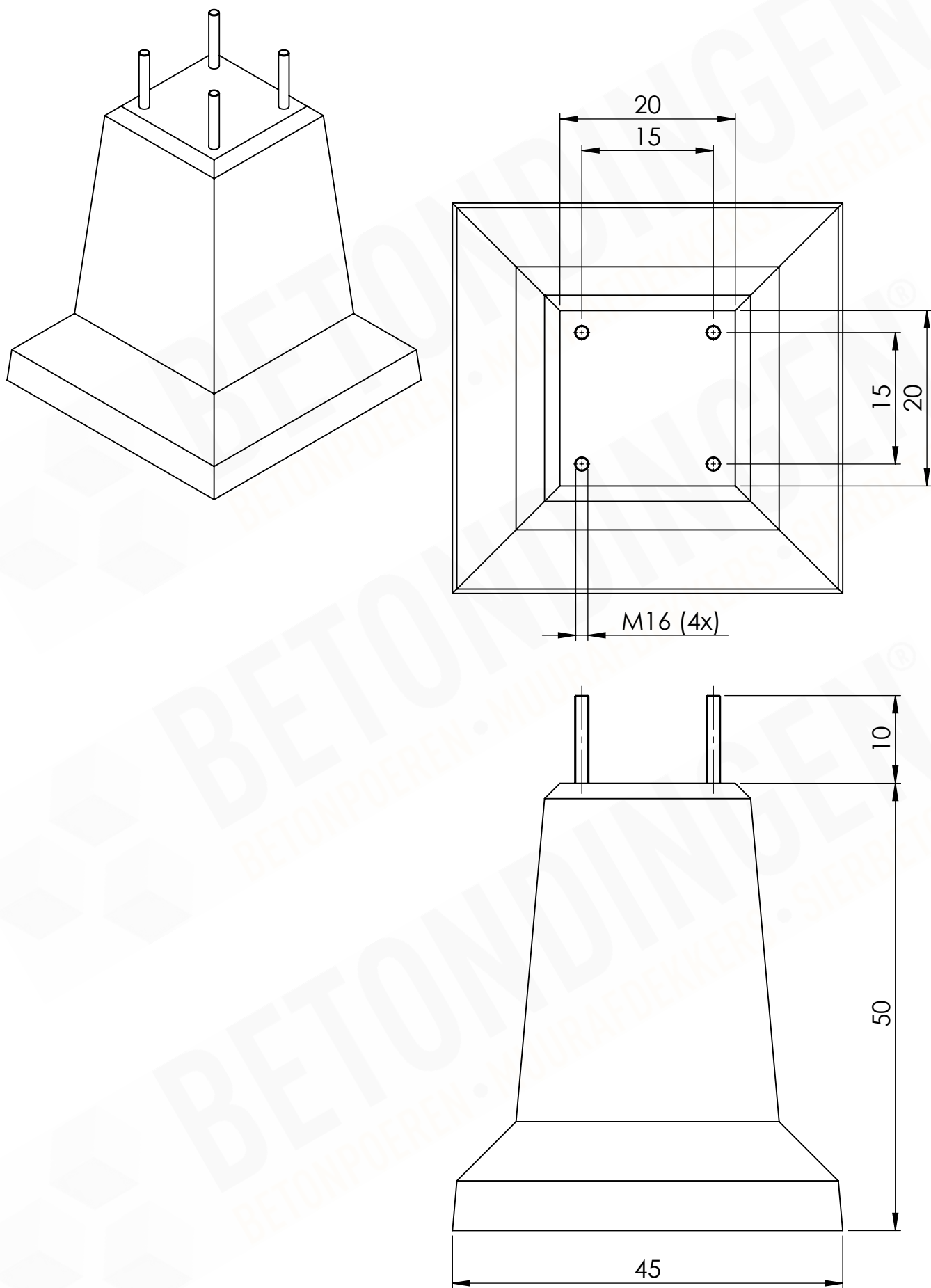
Betonpoer 20x20 en 50 cm hoog grijs 4 keer M16
