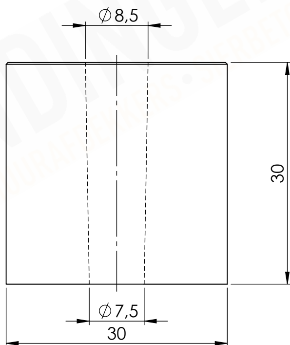
Sokkel / Betonpoer 30x30 en 30 cm hoog grijs met gat diameter 8,5 cm
