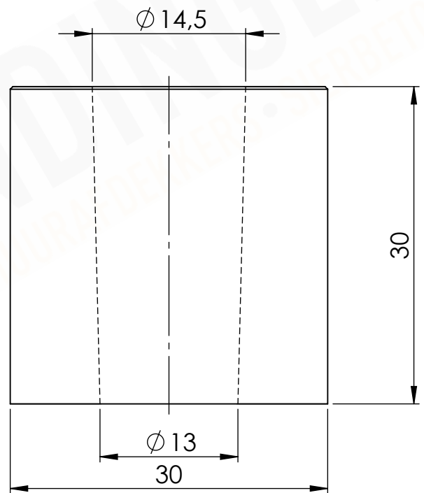
Sokkel / Betonpoer 30x30 en 30 cm hoog grijs met gat diameter 14,5 cm
