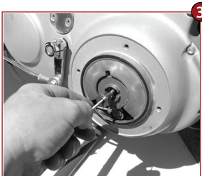
Kupplungsmutter entfernen Remove clutch locknut
