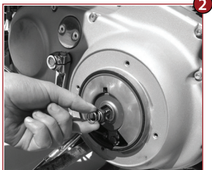
Sicherung entfernen Remove clutch locknut
